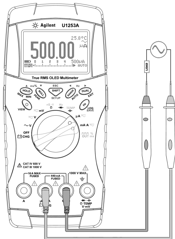
図 2-3 \mu\text{A} および mA 電流の測定
