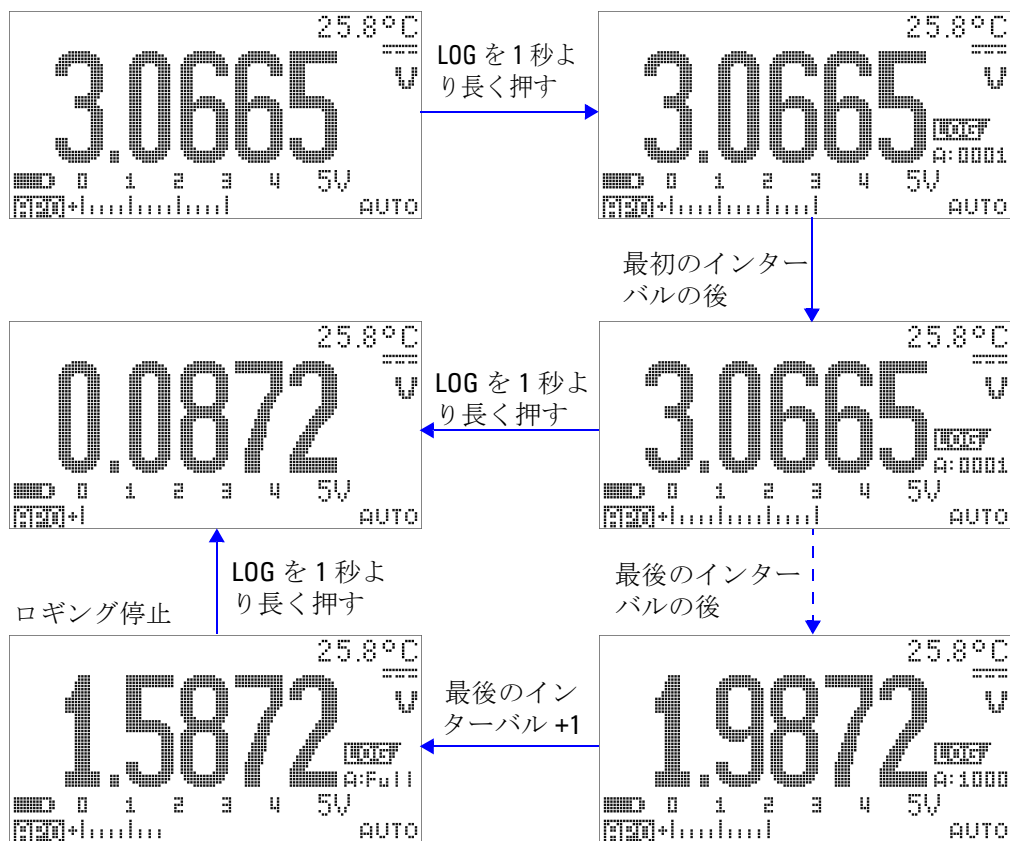
図 3-10 インターバル (タイム) ログイング・モードの動作
