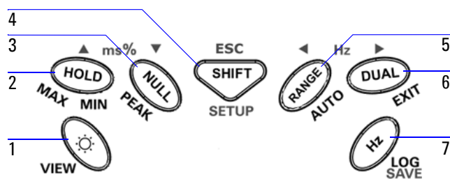
図 1-4 U1253A キーパッド
