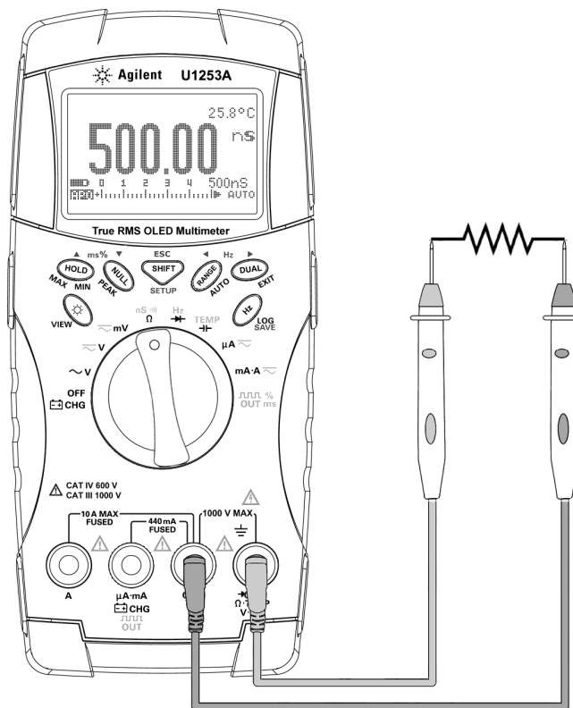
図 2-9 コンダクタンス測定
