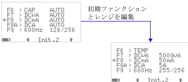
図 4-28 初期測定ファンクション／レンジと初期出力値の編集
