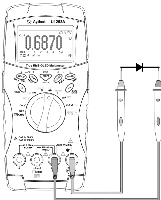
図 2-10 ダイオードの正バイアスの測定
