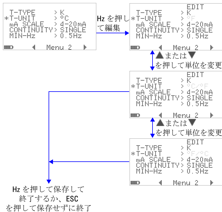
図 4-8 温度単位のセットアップ
