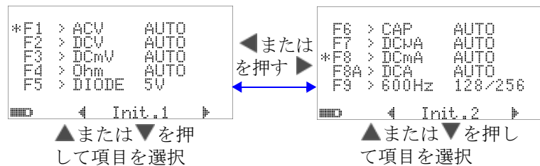
図 4-26 初期ファンクション・ページ間の移動
