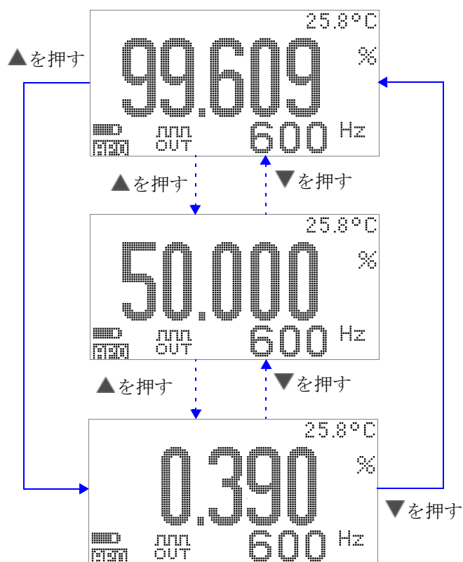
図 3-13 方形波出力のデューティ・サイクル調整
