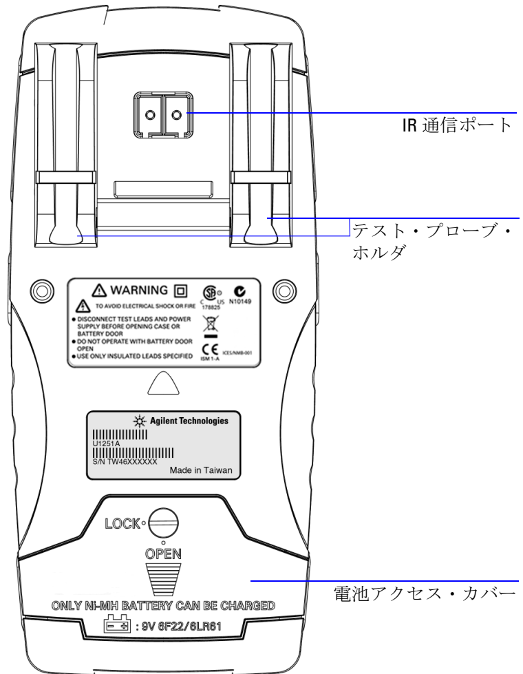
図 1-6 U1253A のリア・パネル
