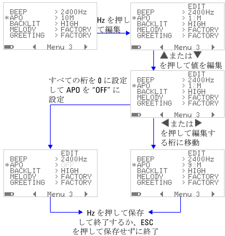
図 4-13 自動省電力機能のセットアップ
