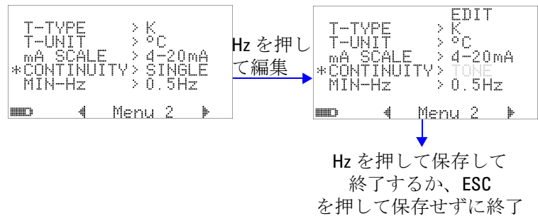
図 4-10 導通テストに使用するサウンドの選択
